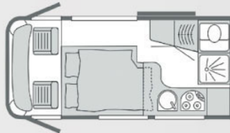
Grundriss Schlagsituation - Duschwanne ausgezogen
