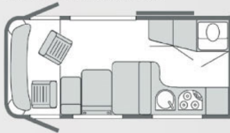
Grundriss Tagsituation mit Tisch in Normalposition
