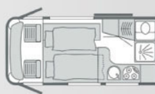
Grundriss Schlagsituation mit optionaler Bettverbreiterung
